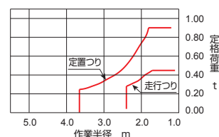
ZAXIS 40UR
