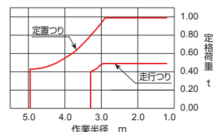
ZAXIS 55UR
