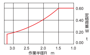
ZAXIS 30UR
