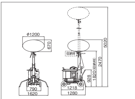
■ 寸法図 [SBL133IDGC] (単位: mm)
