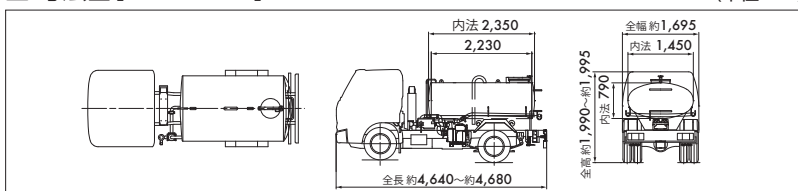
2トン散水車
